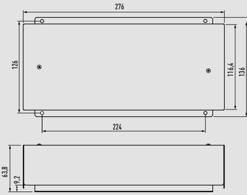
Adattatore comunicazione CZ-CFUNC2
