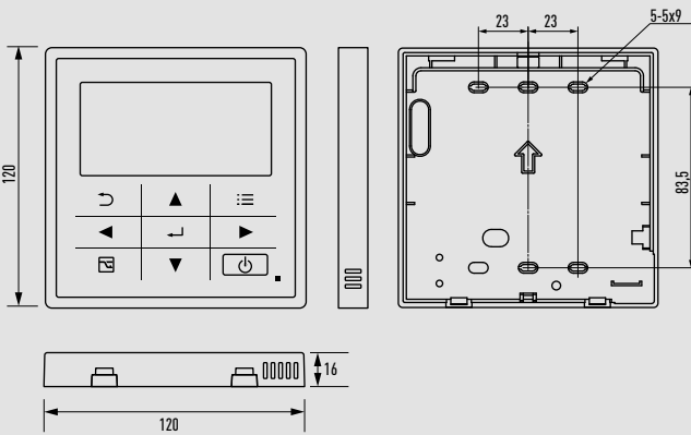
Comando semplificato CZ-RE2C2
