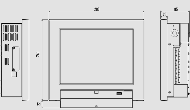
Adattatore locale per controllo ON/OFF CZ-CAPC2
