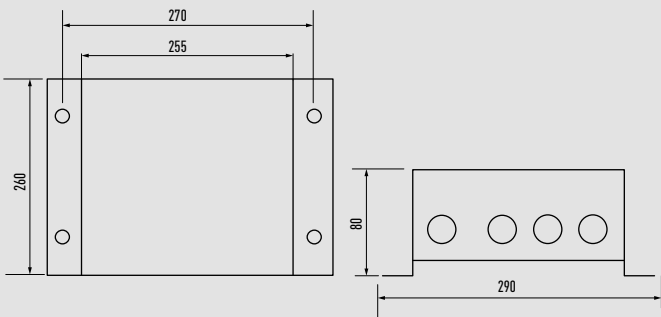
Unità di ingresso/uscita seriale-parallela per unità esterna CZ-CAPDC2
