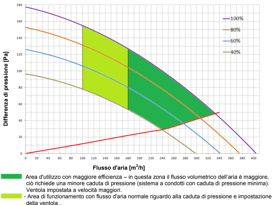
Grafico 1: Caratteristiche aerodinamiche
